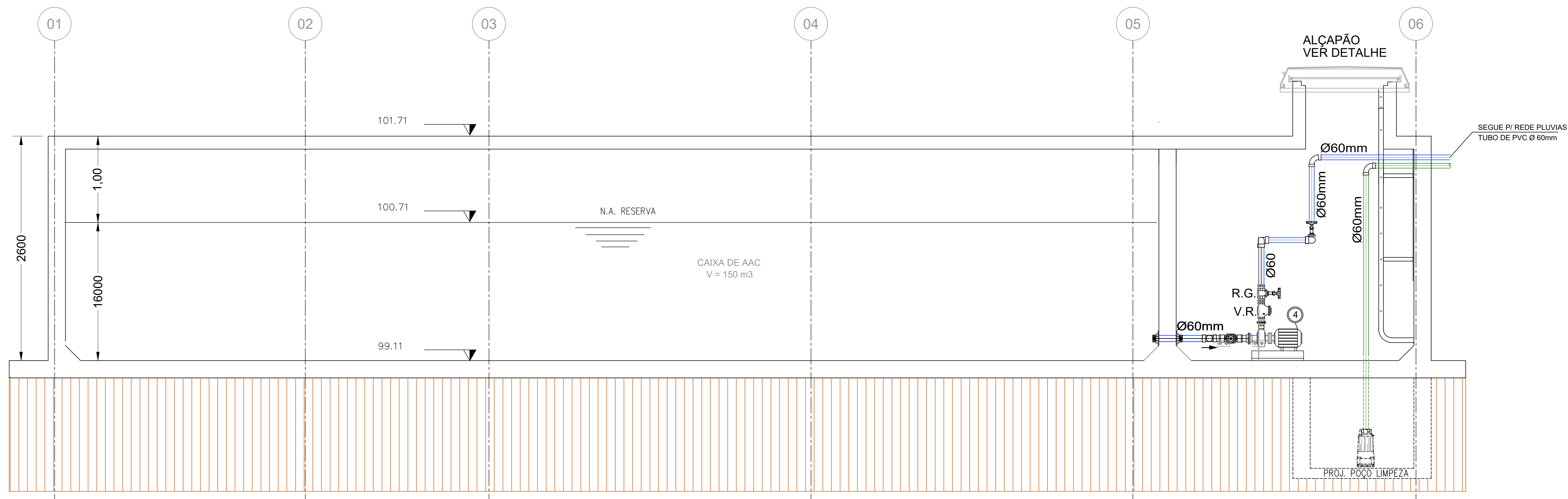
CORTE A-A ESC. 1:25
