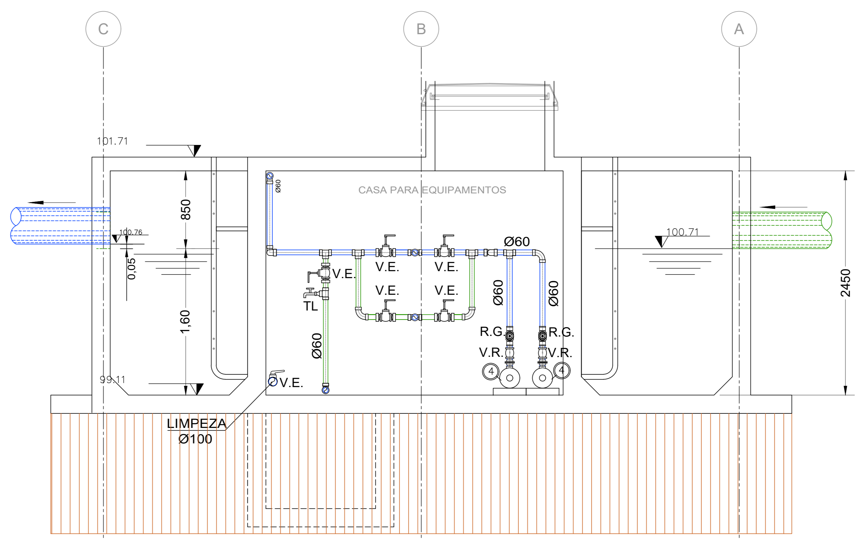
CORTE C-C ESC. 1:25
