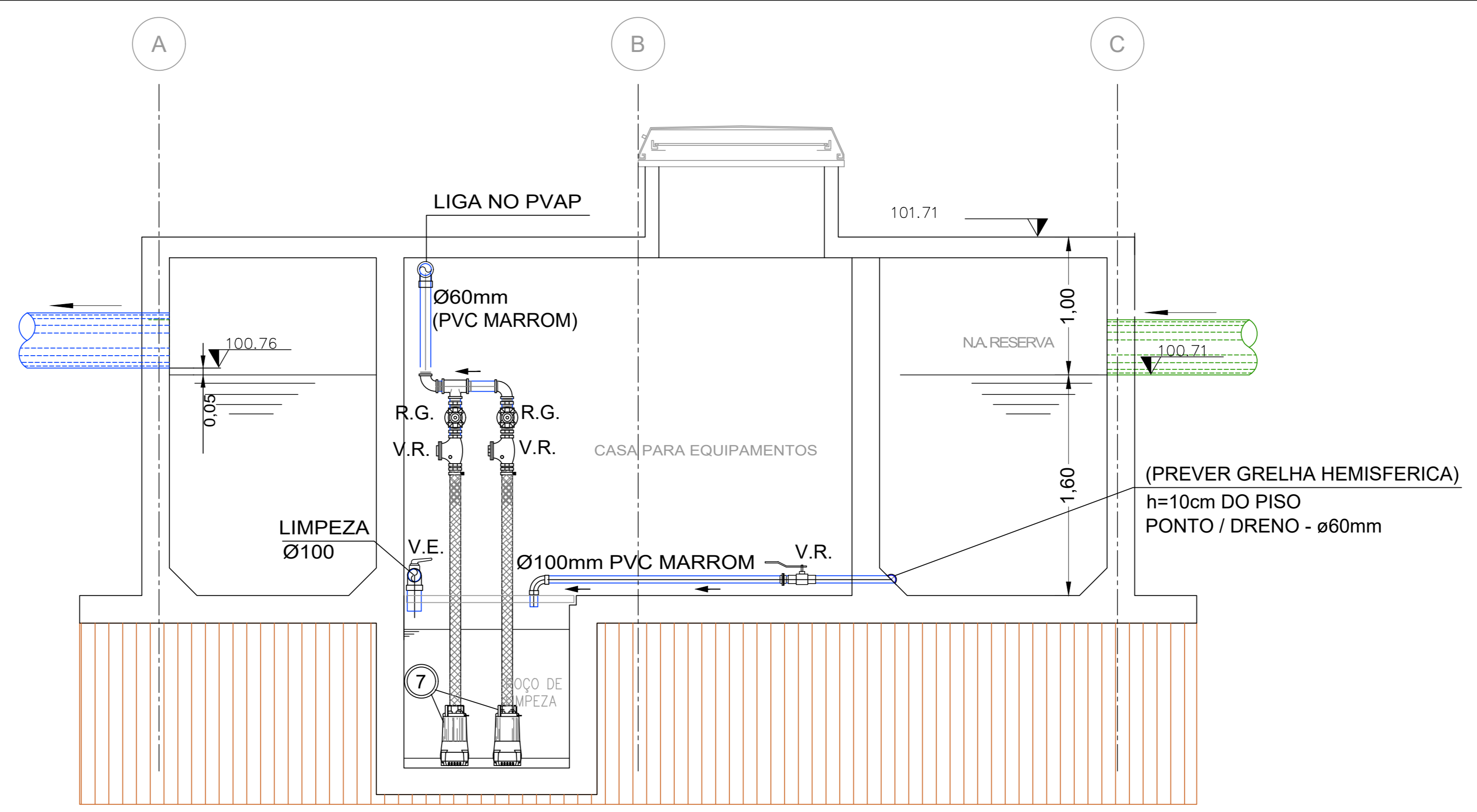
CORTE B-B ESC. 1:25
